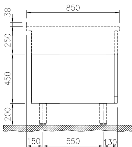
Boven aanzicht
